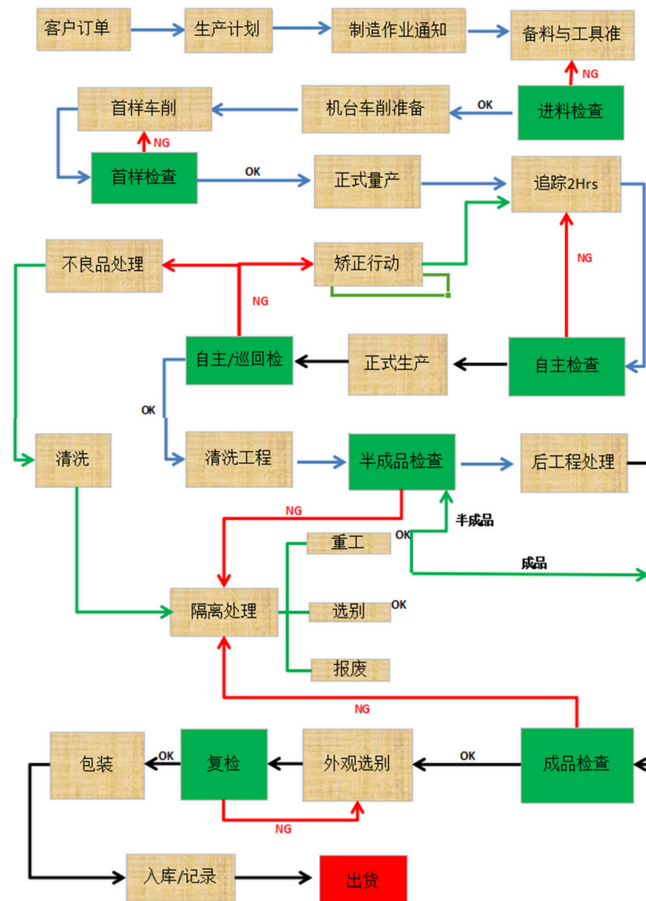
制程流程图
